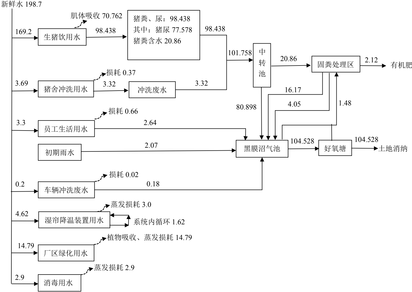
图 3.2-1 项目夏季水平衡图 单位 m³/d
