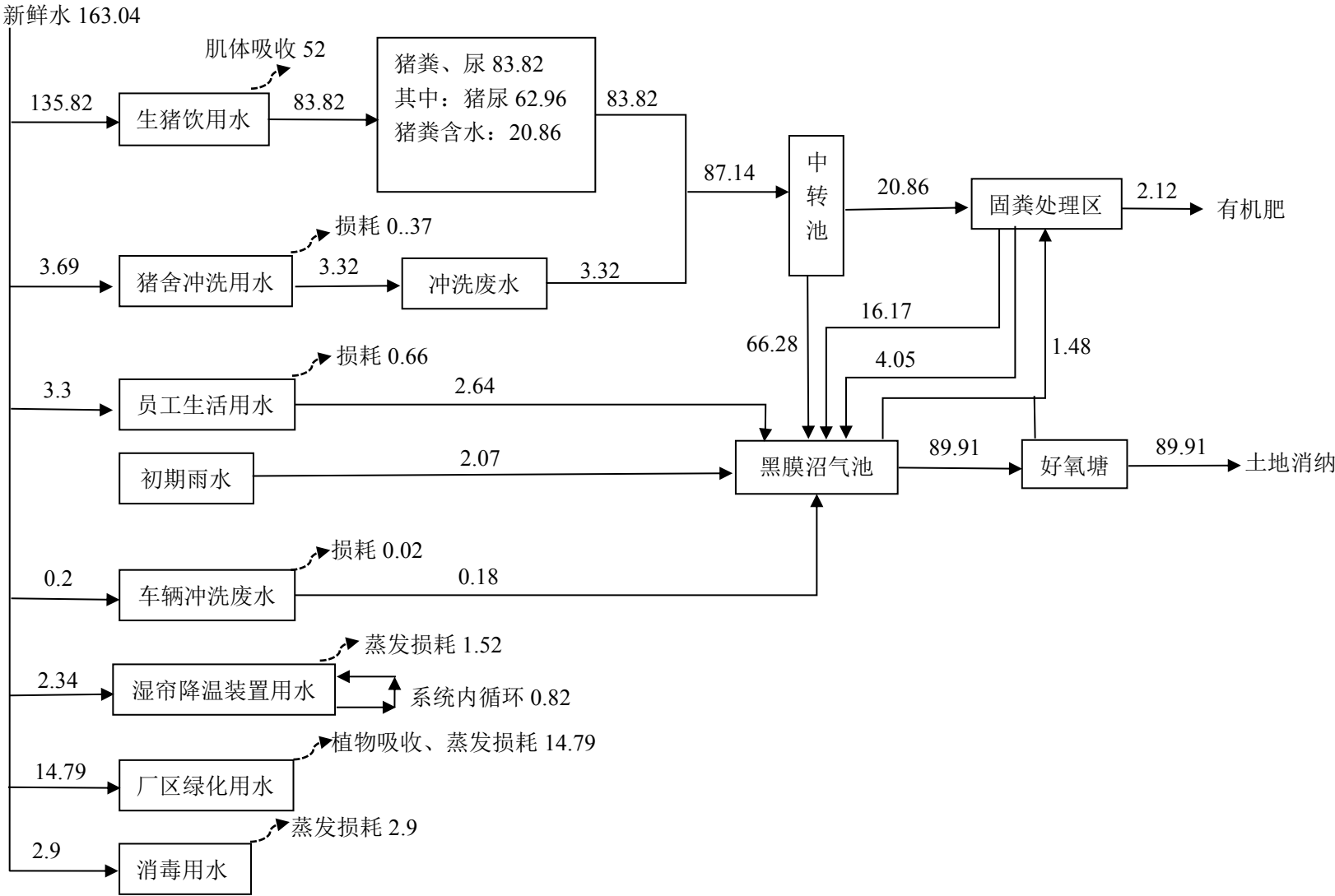
图 3.2-3 项目全年水平衡图 单位 m³/d
