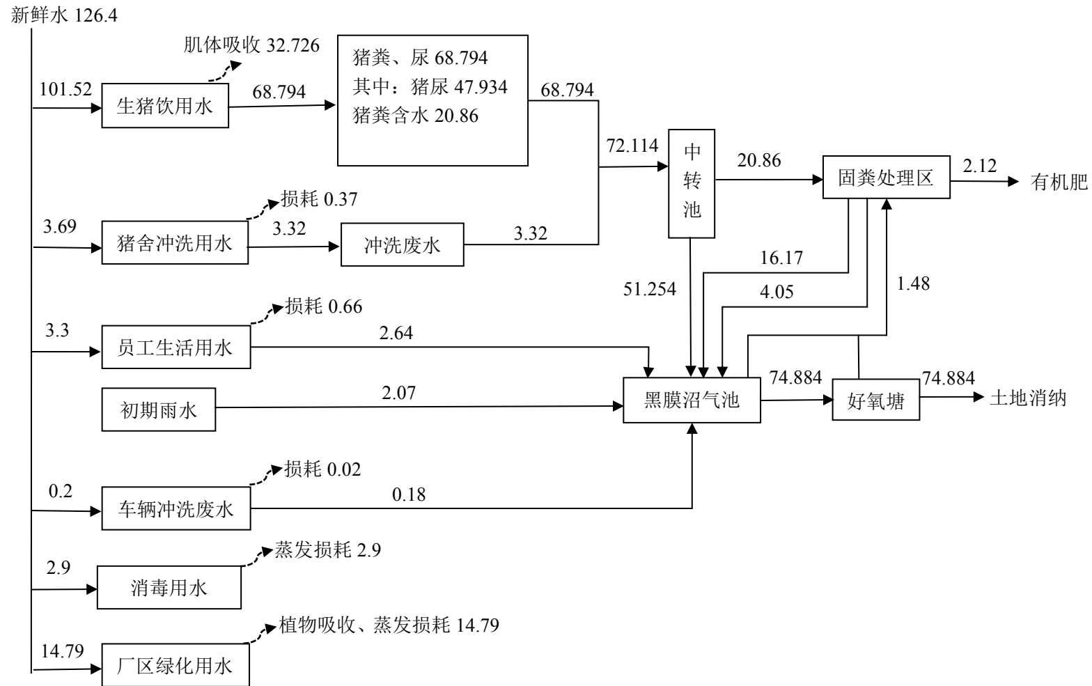
图 3.2-2 项目冬季水平衡图 单位 \text{m}^3/\text{d}
