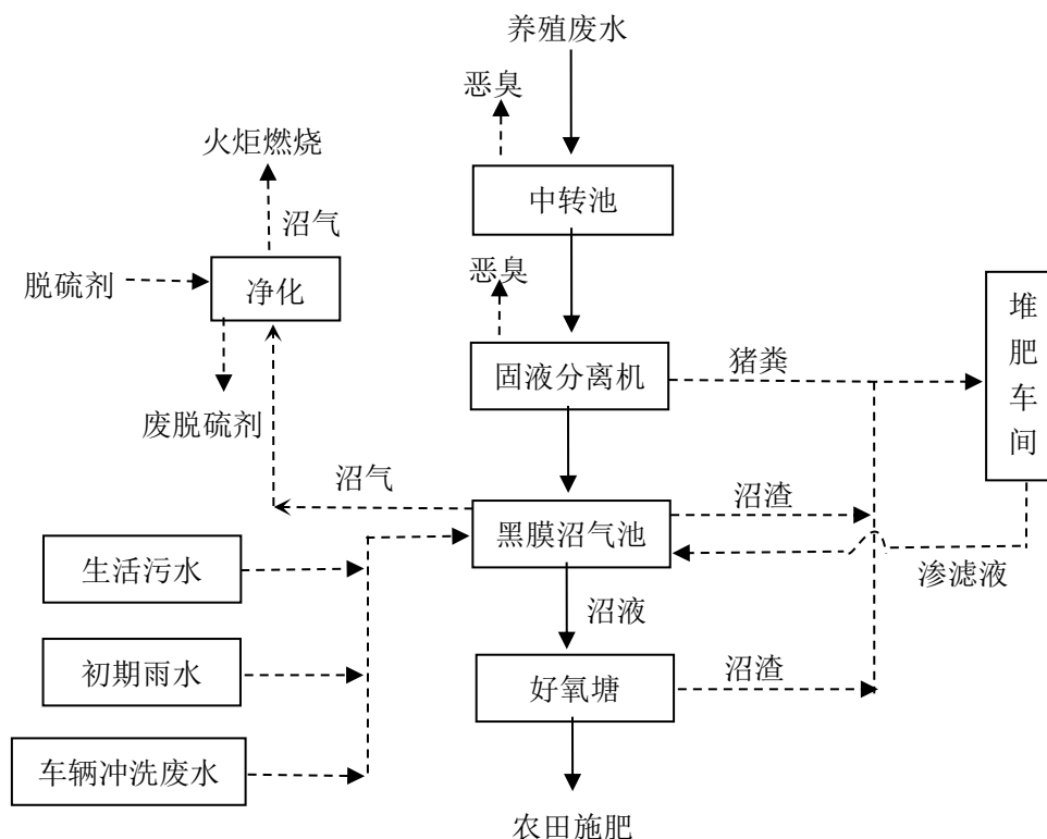
图 6.2-1 污水处理工艺流程图
